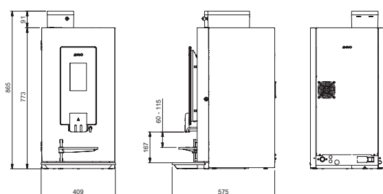
HØJRE SIDEVISNING
