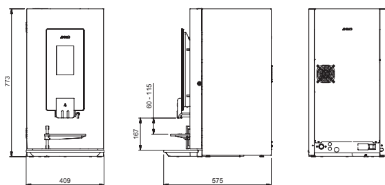
HØJRE SIDEVISNING
