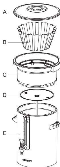
Container + toebehoren koffie Fig. 6
