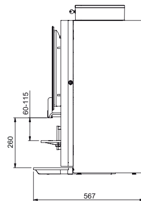
ZIJAAANZICHT RECHTS
