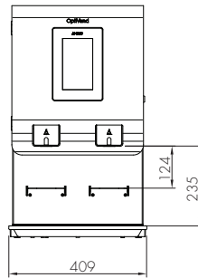
OPTIVEND TS HS DUO TOUCH ZIJAAANZICHT Alle afmetingen in mm.
