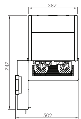
BOVENAANZICHT
