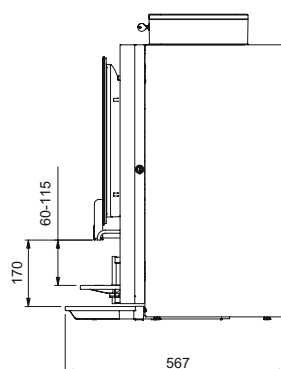
WIDOK Z BOKU – PRAWA STRONA
