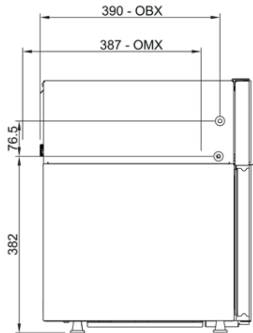
Ansicht von links
