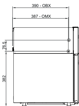
LINKER ZIJAAZICHT
