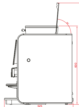
SEITENANSICHT RECHTS
